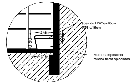
DETALLE BANCOS Esc: 1:50
