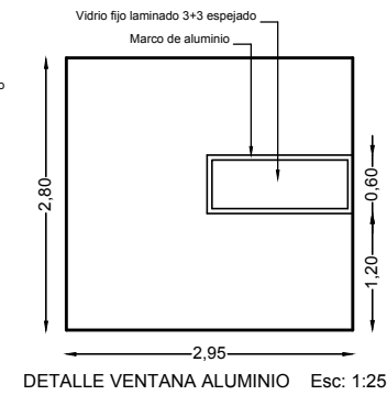
DETALLE VENTANA ALUMINIO Esc: 1:25
