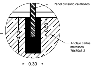
DETALLE ANCLAJE PANEL DIVISORIO Esc: 1:25
